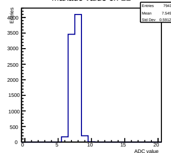
Maxadc value ch 11
