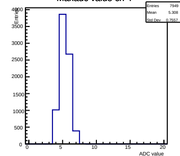
Maxadc value ch 4
