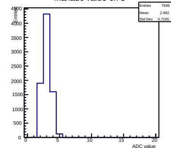
Maxadc value ch 8
