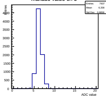
Maxadc value ch 5
