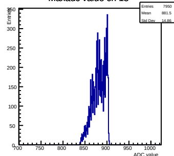
Maxadc value ch 13
