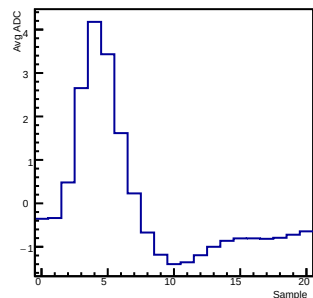
Maxadc value ch 8
