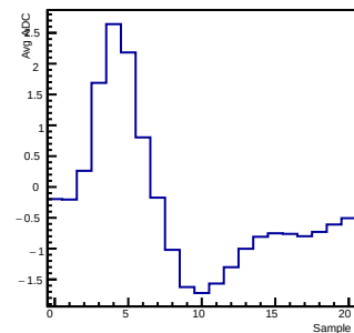
Maxadc value ch 15
