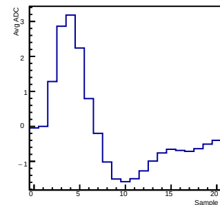
Maxadc value ch 11
