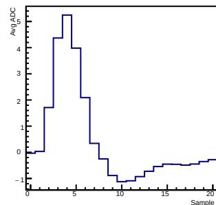
Maxadc value ch 9
