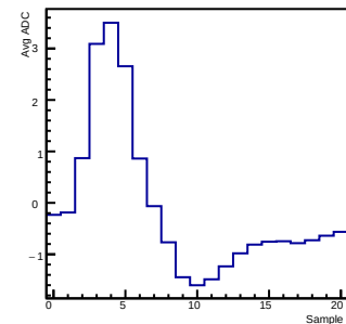
Maxadc value ch 7
