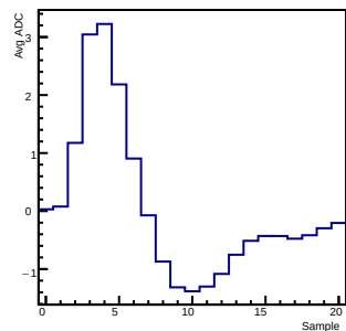
Maxadc value ch 12
