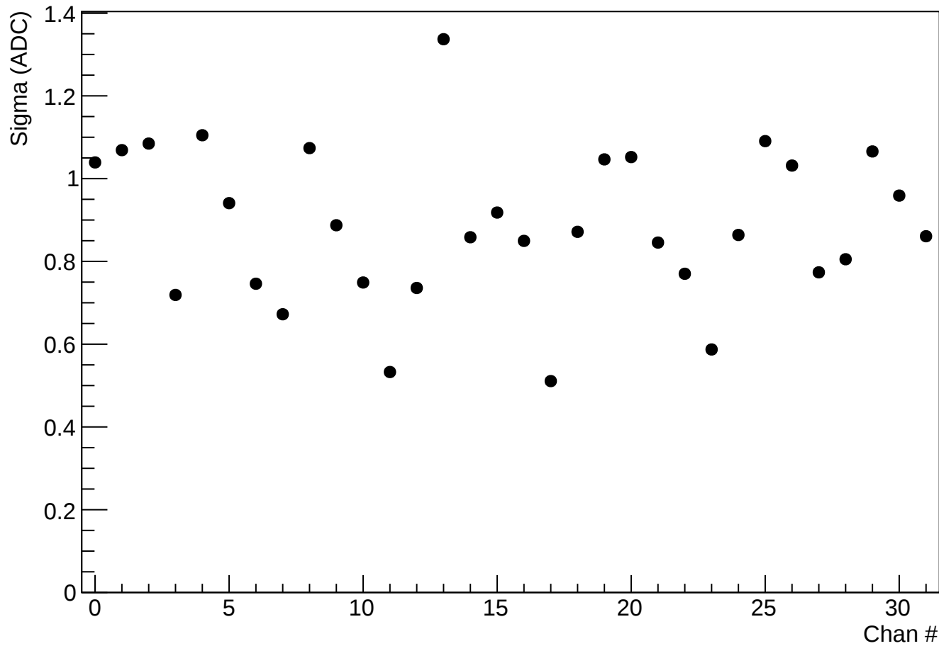
ns_vs_chNo
