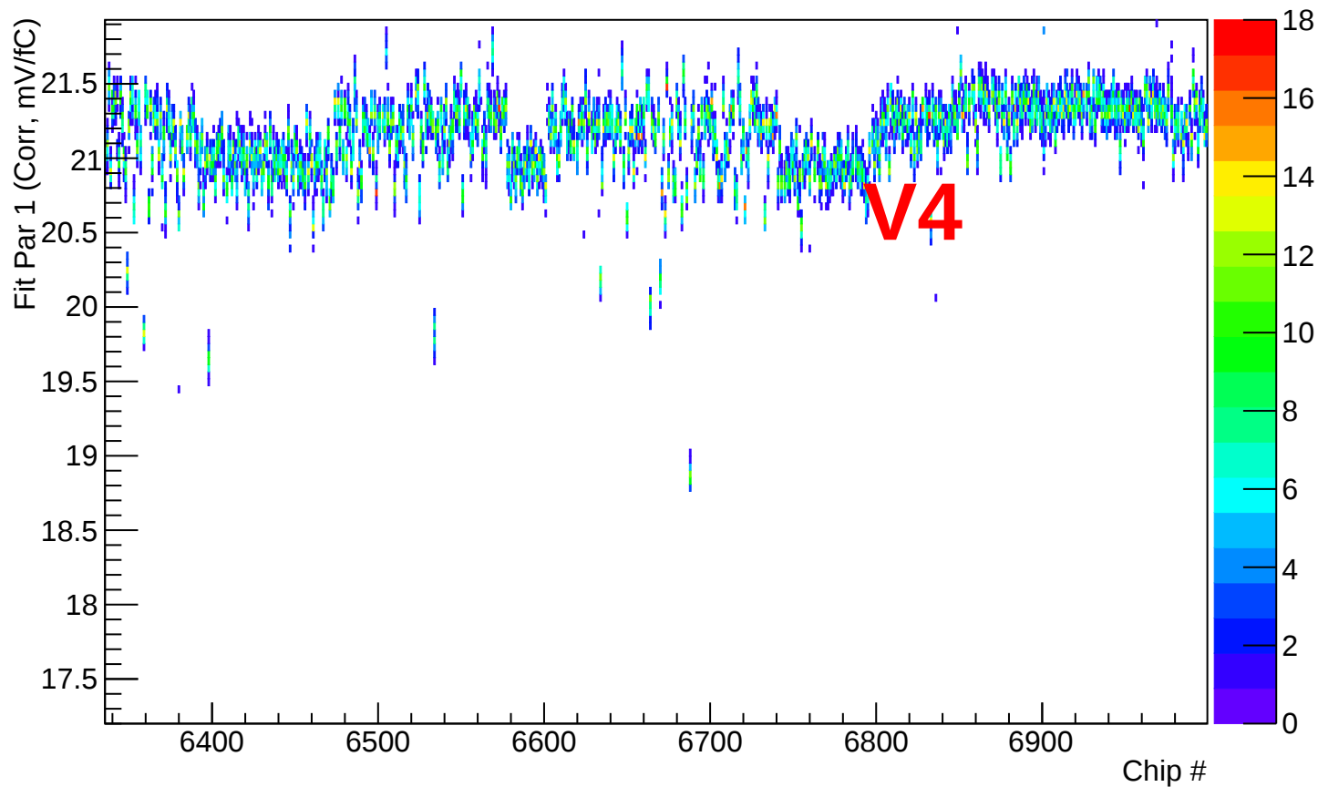
Fit Par 1 (Corr, mV/fC) vs Chip #
